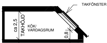
SEKTION A-A
