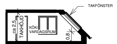
SEKTION A-A
