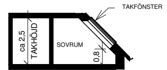
SEKTION A-A
