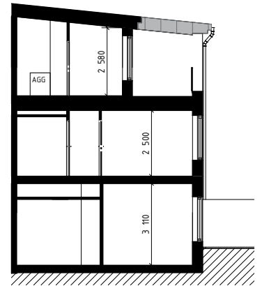
SEKTION
