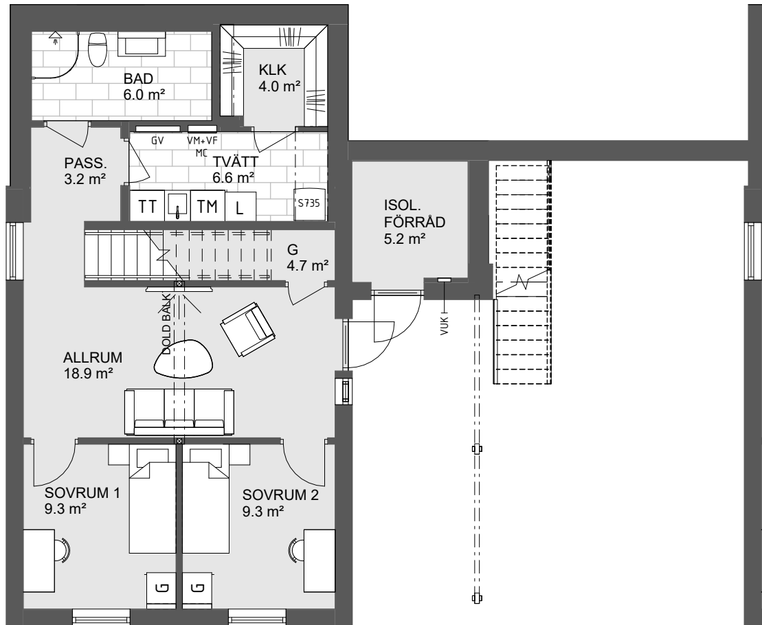
BOTTENVÅNING
