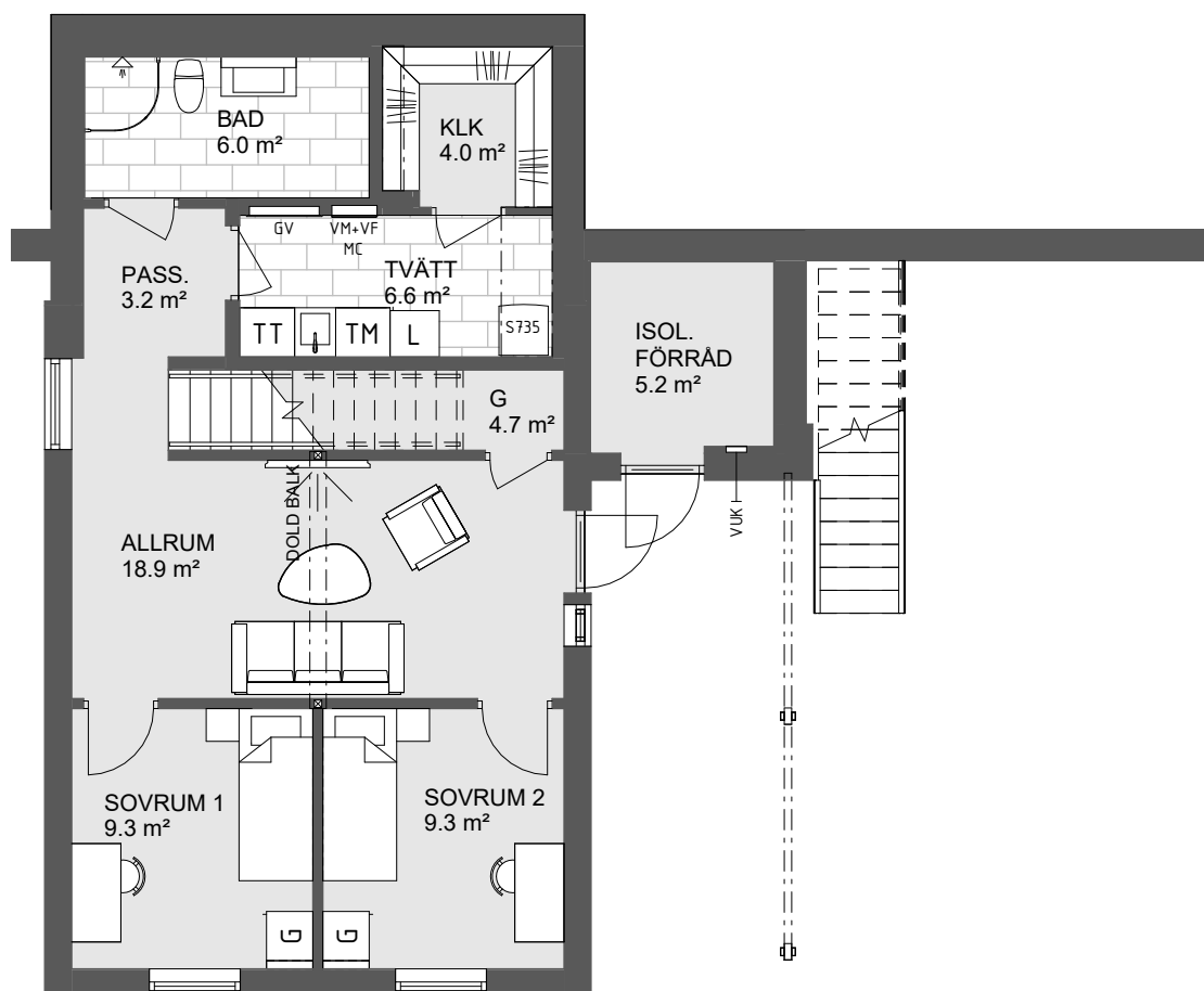
BOTTENVÅNING
