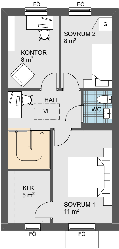
↑ Planlösning övre plan, tillval vägg.
