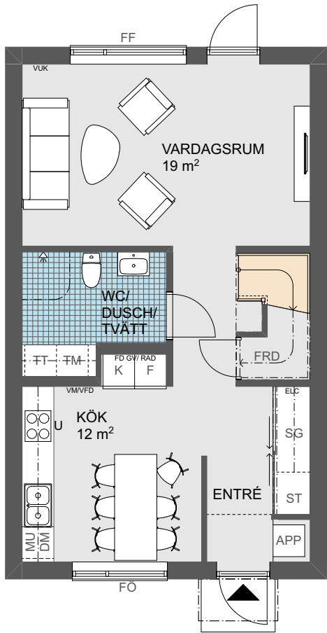
↑ Planlösning gavel vänster.
