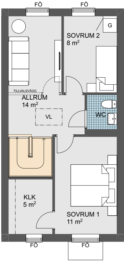
↑ Planlösning övre plan, standard.
