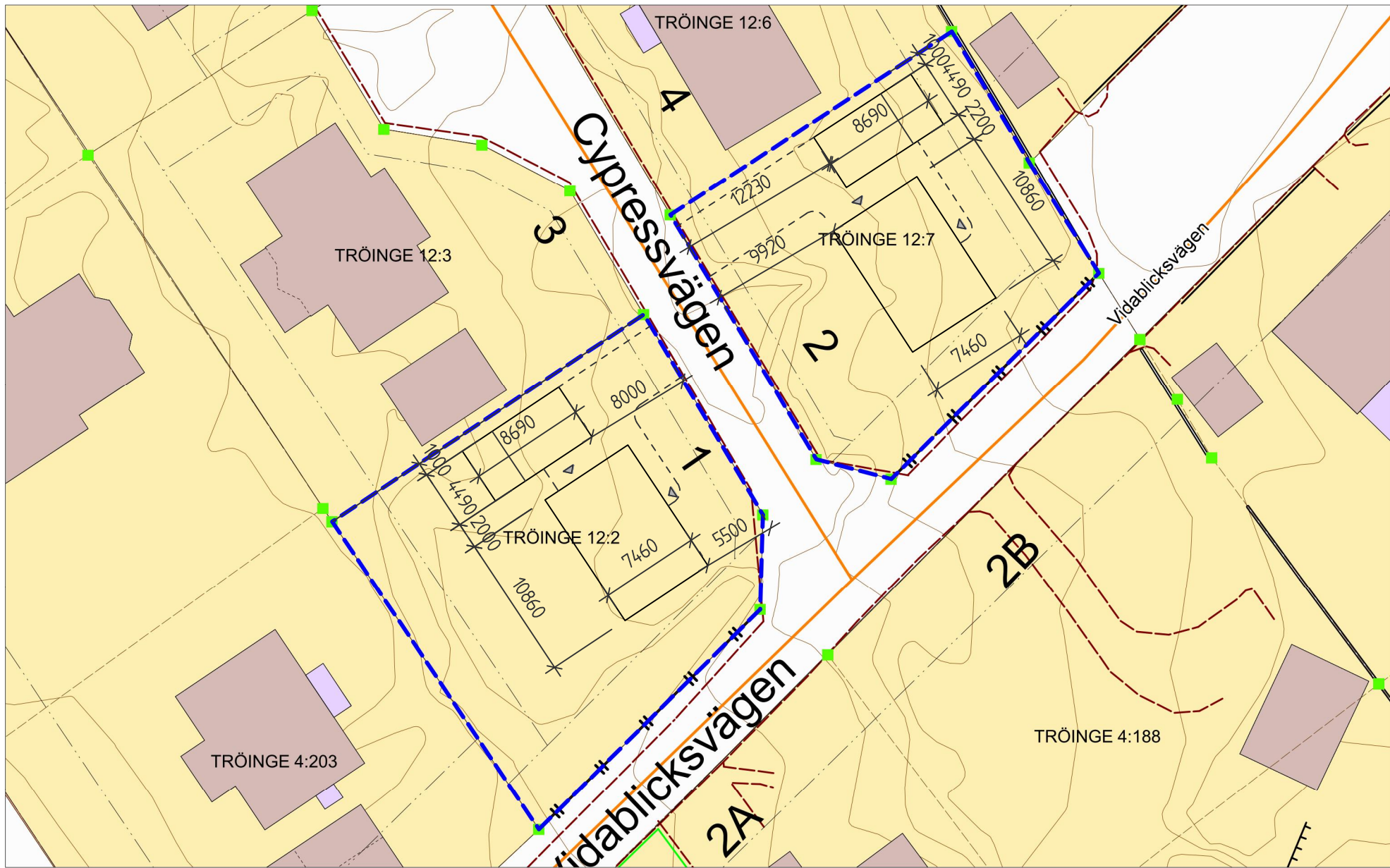
A4 SKALA 1:400
