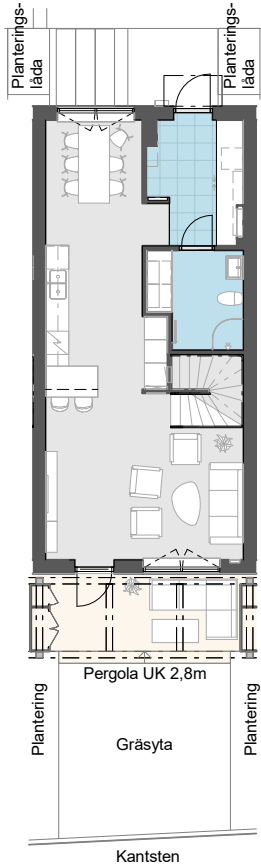
PLAN 1 ÖVERSIKT (HALVSKALA)
