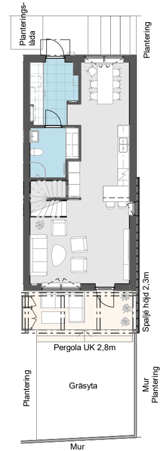
PLAN 1 ÖVERSIKT (HALVSKALA)
