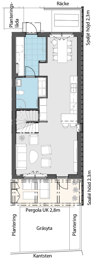
PLAN 1 ÖVERSIKT (HALVSKALA)
