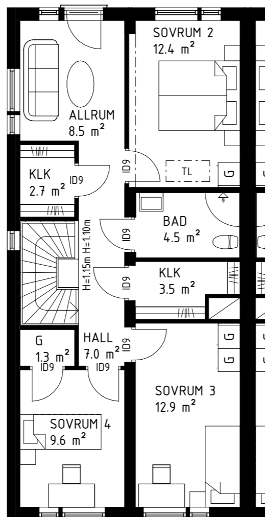
Hustyp 137 Övervåning Alternativ A: Allrum + Klädskammare
