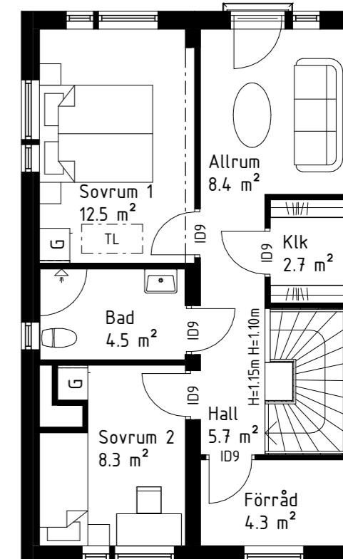
Hustyp 107 Övervåning Alternativ B: Allrum + Förråd
