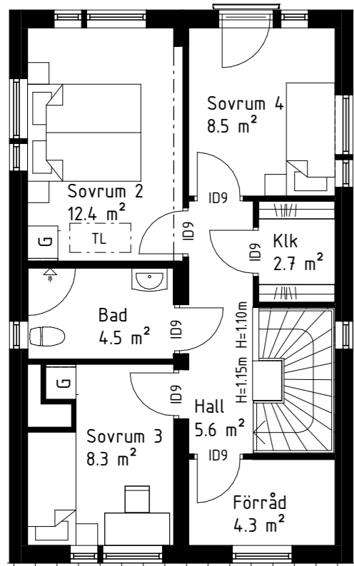
Hustyp 120 Övervåning Alternativ D: Sovrum 4 + Förråd
