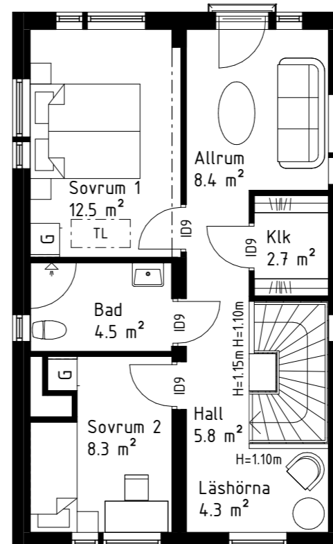
Hustyp 107 Övervåning Alternativ A: Allrum + Läshörna
