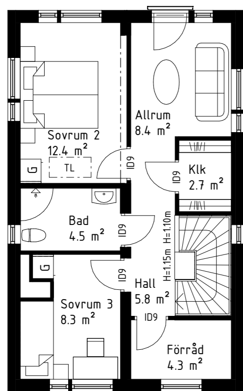
Hustyp 120 Övervåning Alternativ B: Allrum + Förråd
