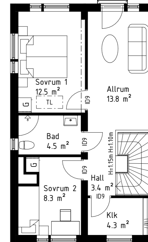
Hustyp 107 Övervåning Alternativ E: Stort Allrum ist. för Klädskammare och Klädskammare istället för Läshörna
