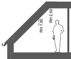
SEKTION A-A
