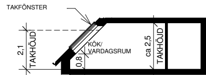
SEKTION A-A
