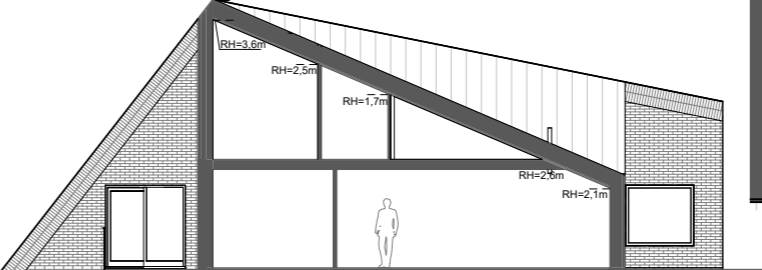
Sektion A-A (halvskala)
