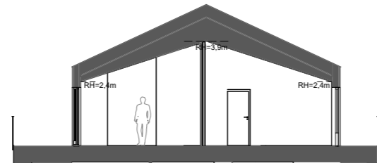
Sektion A-A (halvskala)
