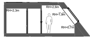
Sektion A-A (halvskala)
