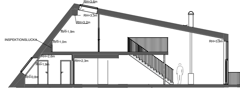
Sektion B-B (halvskala)
