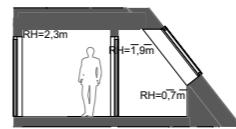
Sektion B-B (halvskala)
