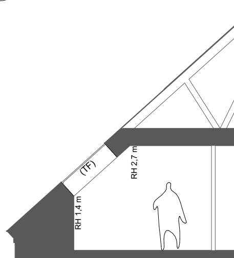
Vindssektion, snedtak
