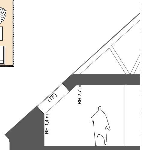
Vindssektion, snedtak
