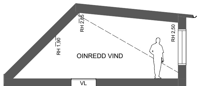
SEKTION B-B
