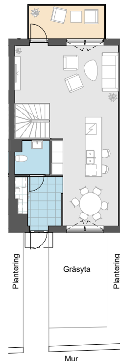
PLAN 1 MED ENTRÉYTA (HALVSKALA)
